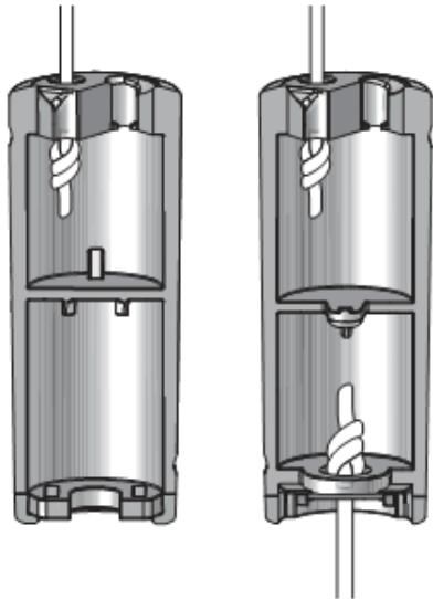
Product met 2 optrekkorden
